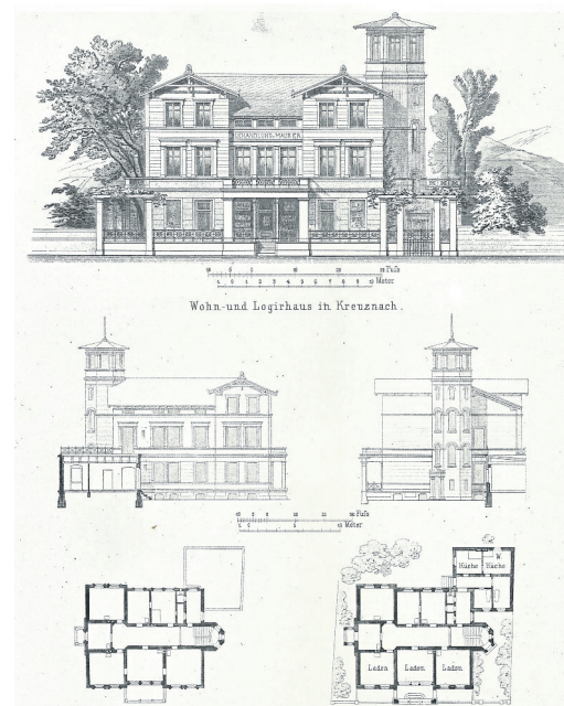
Entwurf des Wohn- und Logierhauses.
